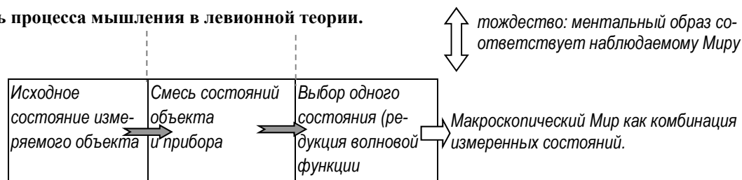
Рис. 8. Схема процесса квантового измерения.
